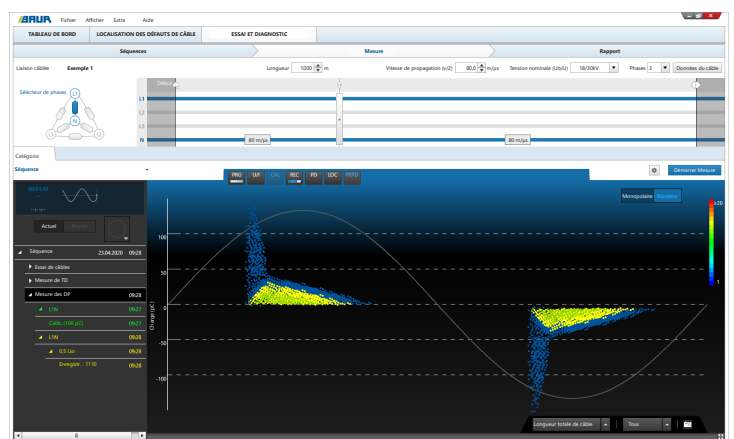
Exemple : Mesure des DP – Représentation des DP avec positionnement de phase (PRPD)
